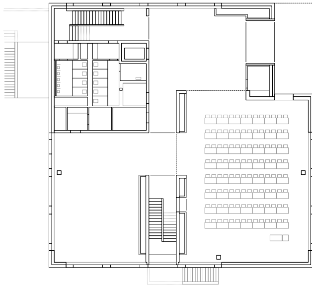
Grundrisse EG; 1. OG
