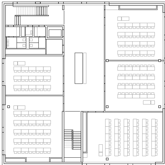
Grundrisse 2. und 3. OG, Schnitt
