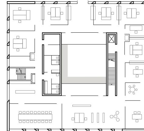
Grundriss OG
