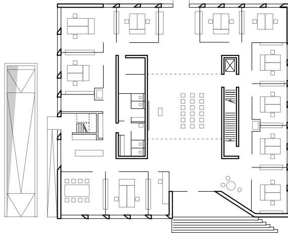
Grundriss EG
