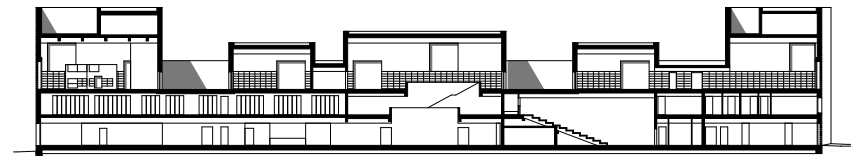
Längsschnitt
