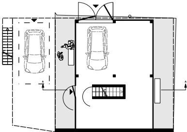
EG, M 1:300
