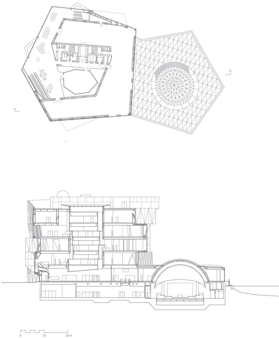
Grundrisse 1. OG, Schnitt, 1:1000
