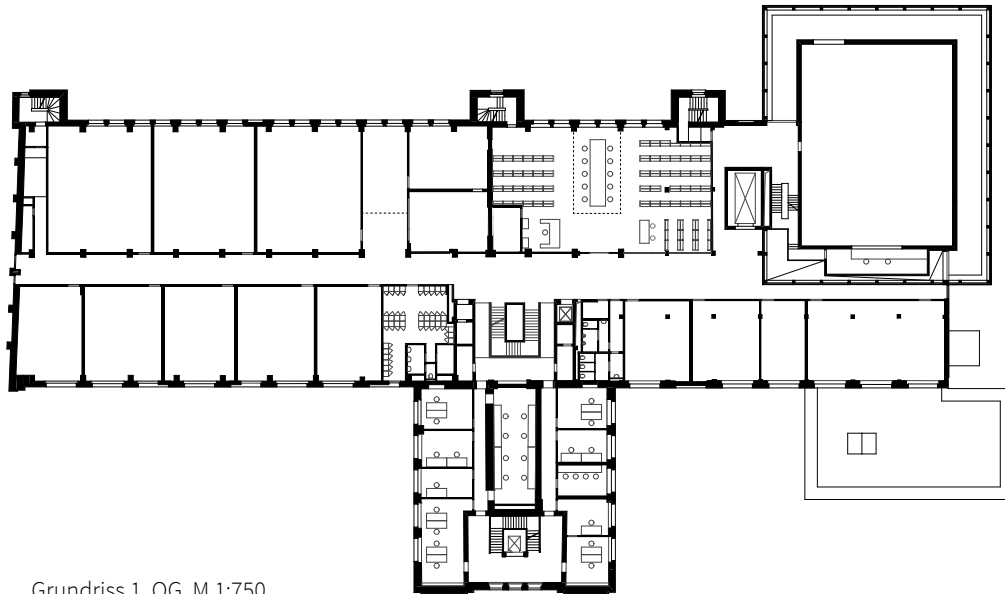
Grundriss 1. OG, M 1:750
