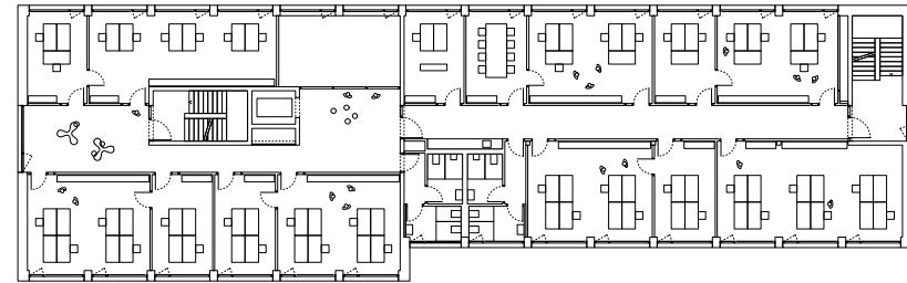
Grundriss 1. OG, M 1:500
