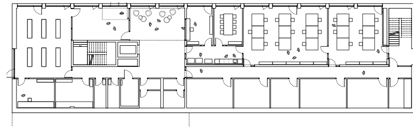
Grundriss Erdgeschoss, M 1:500
