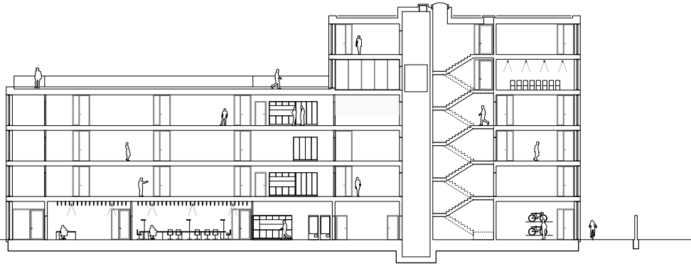
Längsschnitt, M 1:500
