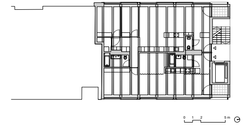
Grundriss 4. OG, M 1:500
