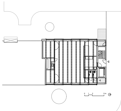
Grundriss EG, M 1:500
