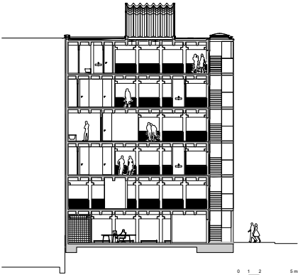
Längsschnitt, M 1:500
