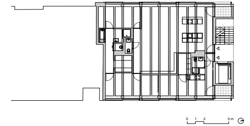
Grundriss 5. OG, M 1:500
