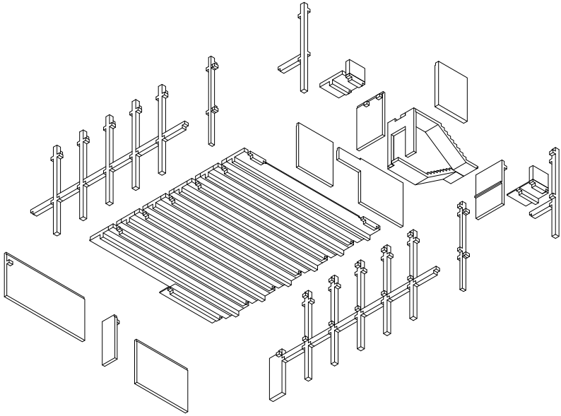
Explosionsaxonometrie
