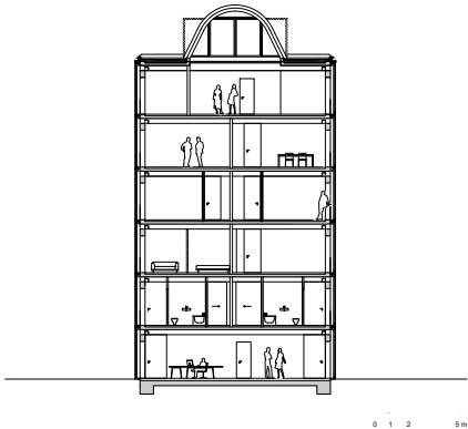
Querschnitt, M 1:500
