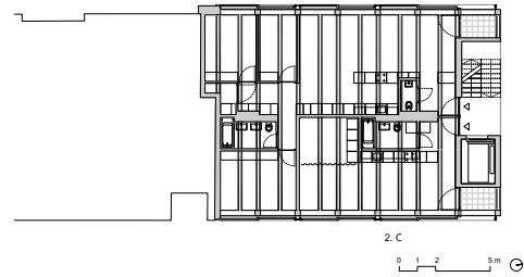
Grundriss 2. OG, M 1:500
