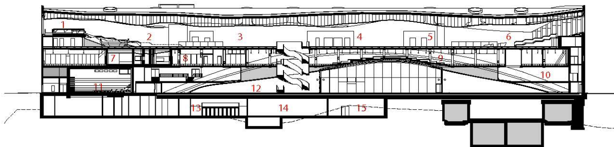
Längsschnitt, 1:1000
