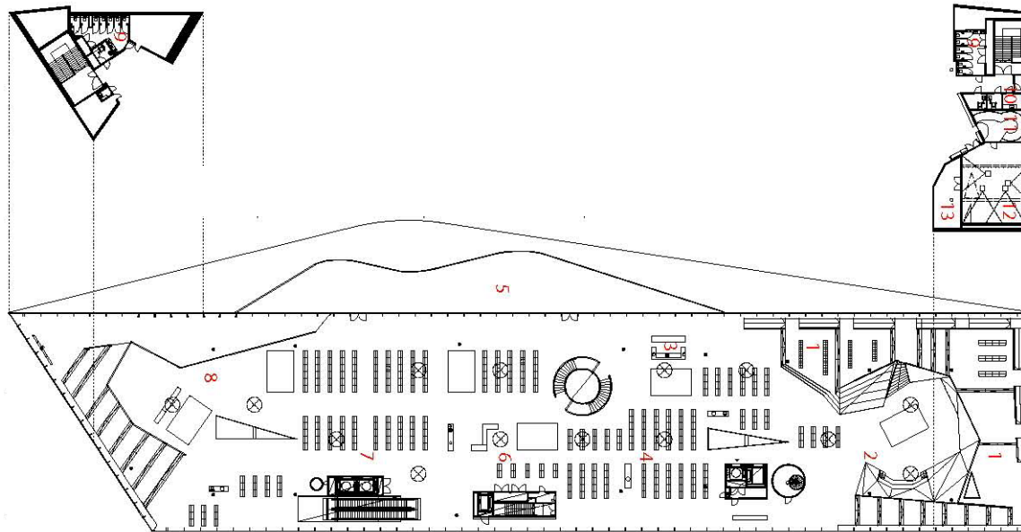
3. Obergeschoss, M 1:1000
