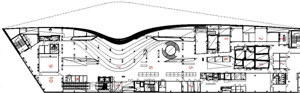
1. Obergeschoss, M 1:1000
