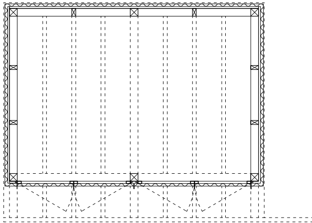
Grundriss
