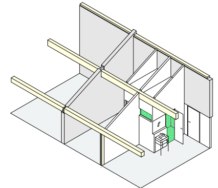
Axonometrie Zimmer OG
