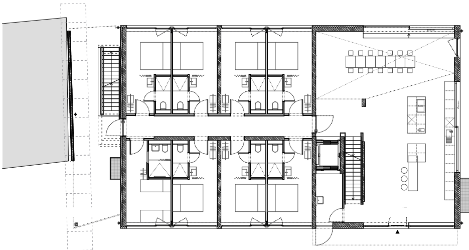
Grundrisse EG, OG, M 1:250
