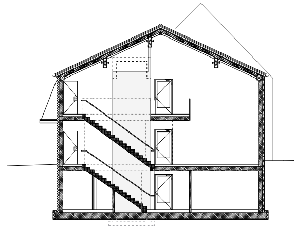
Querschnitt, M 1.250
