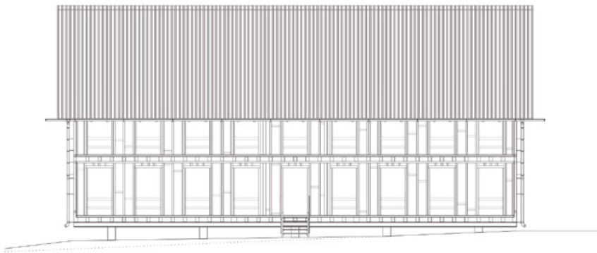
Ansicht Ost, 1:200
