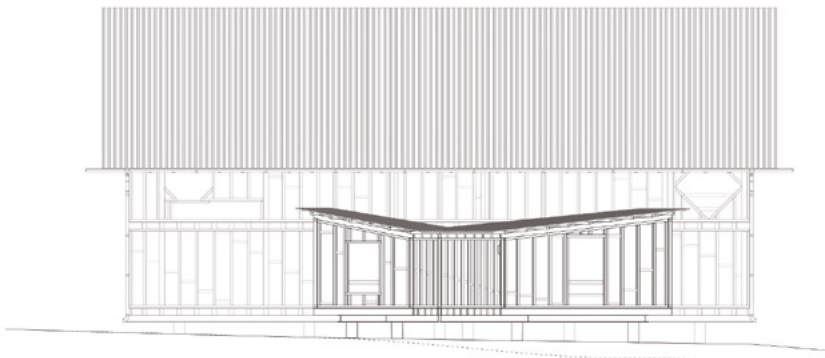
Ansicht West, 1:200
