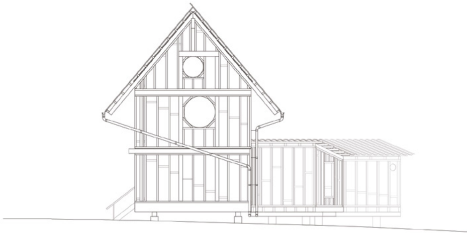
Ansicht Nord, 1:200
