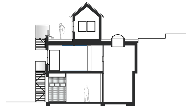
Schnitt neu, 1:500
