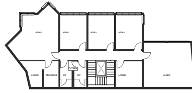
Grundriss OG Bestand, 1:500
