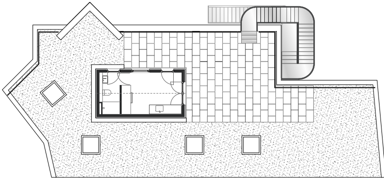
Grundriss DG neu, 1:250
