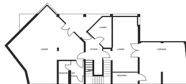
Grundriss EG Bestand, 1:500
