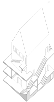
Umlaufende Erschließung in der Fuge zwischen Alt und Neu
