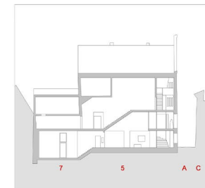
Längsschnitt Seitenflügel Museum / Treppe Süd / Foyer
