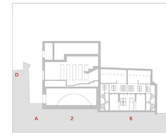
Längsschnitt Theater / Ganghaus
