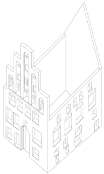
Bestand Denkmalschutz: Fassaden und Außenmauerwerk
